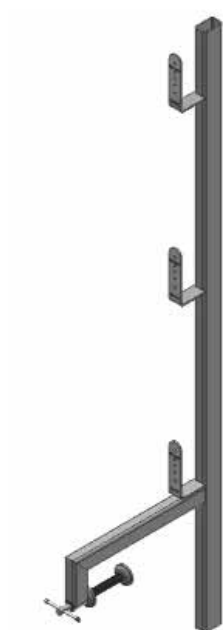
Fig. 9.1.2.1.1-1 Parapetto provvisorio ammorsato con ganascia fissa
