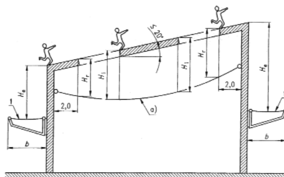
Fig. 9.2.1-1 Altezze di caduta consentite e larghezze di raccolta richieste per zone di lavoro inclinate tra 0^\circ e 20^\circ
