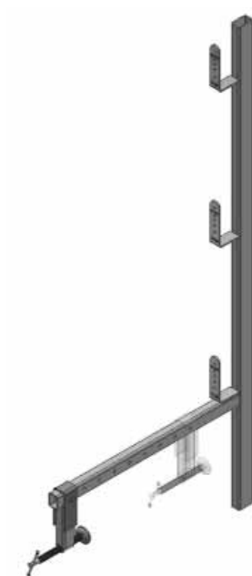
Fig. 9.1.2.1.1-2 Parapetto provvisorio ammorsato con ganascia regolabile
