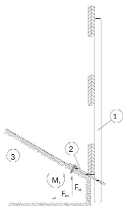
Fig. 8.1-1 Esempio di reazioni vincolari relative alle azioni statiche
