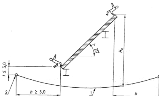
Fig. 9.2.1-1 Altezze di caduta consentite e larghezze di raccolta richieste per zone di lavoro inclinate tra 0^\circ e 20^\circ
