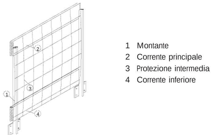
Fig. 6.1-2 Parapetto provvisorio con protezione intermedia
