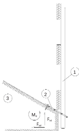
Fig. 8.1-2 Esempio di reazioni vincolari relative alle azioni dinamiche
